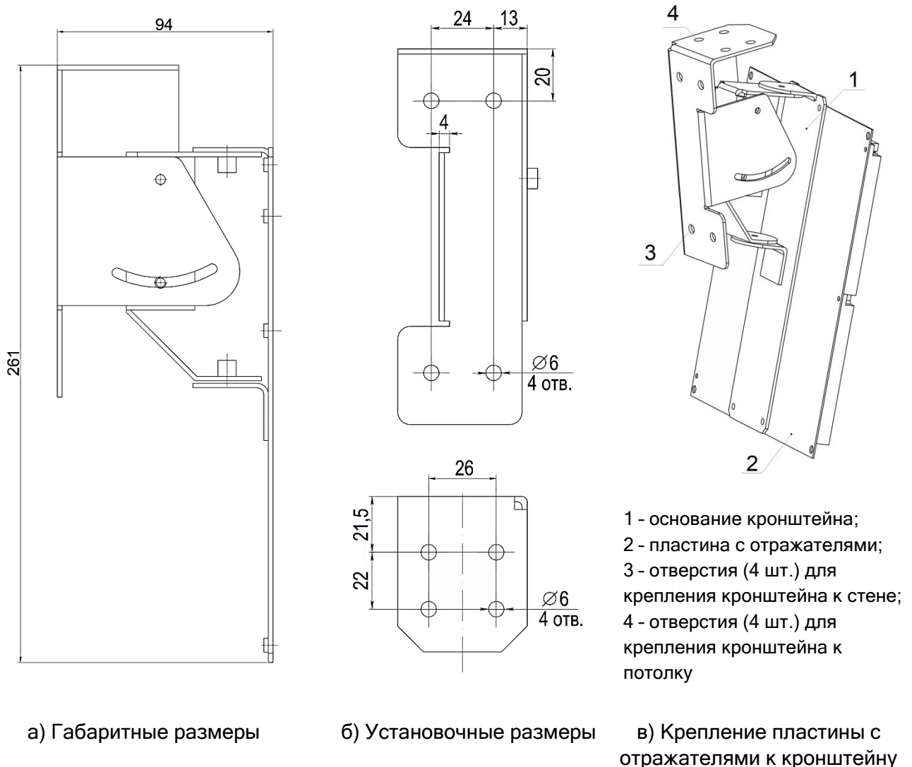
Рисунок 1 - Общий вид кронштейна
